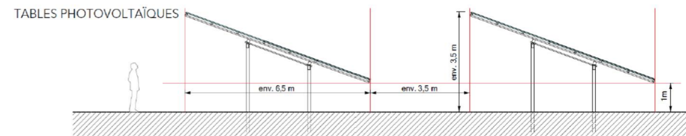
Figure 40 : Vue en coupe d'une table photovoltaïque en pieux (Source : Photosol)
